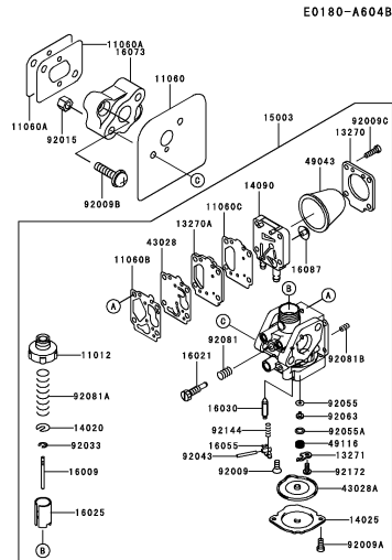
B-09 CARBURETOR
